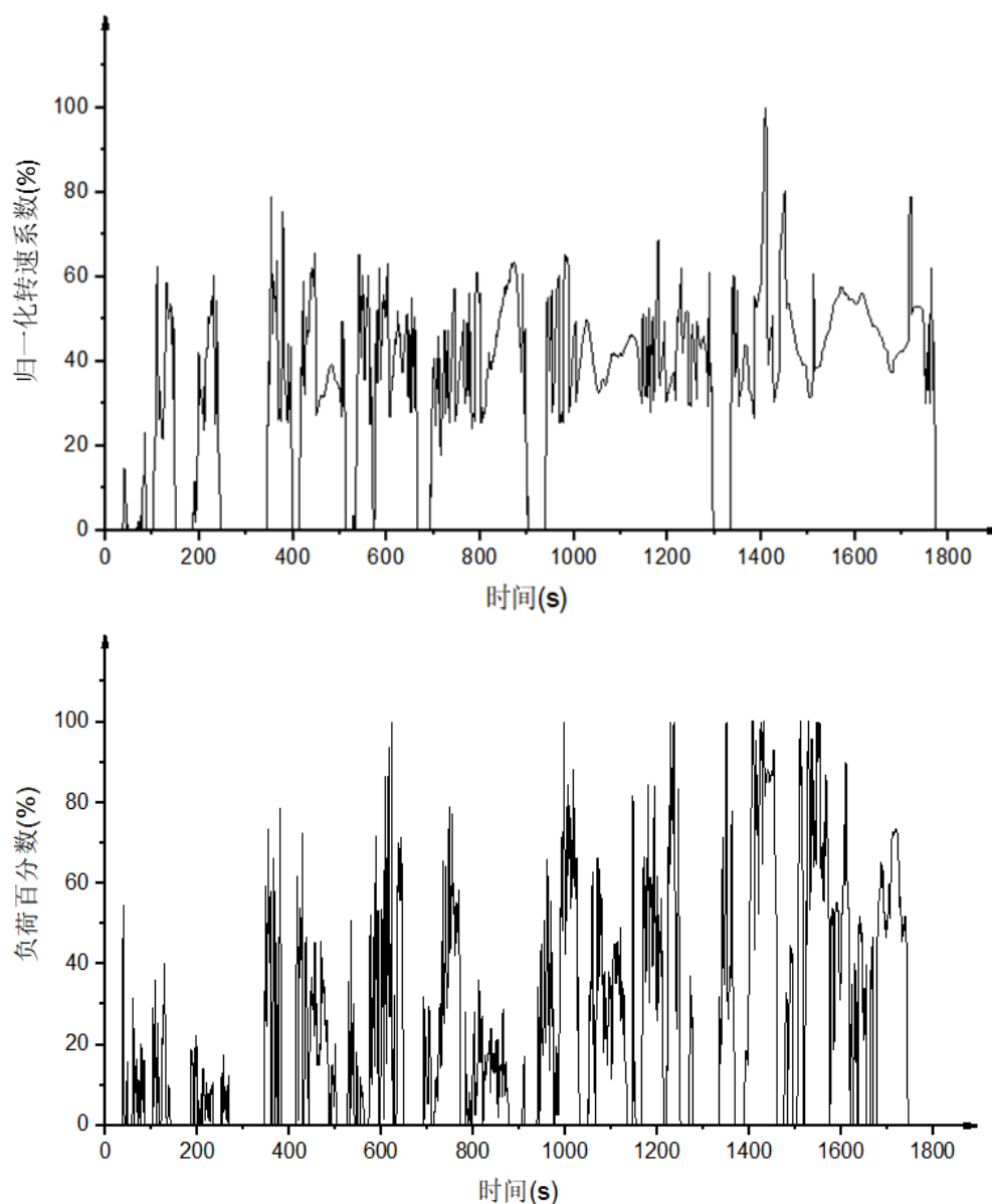
图 1 中国发动机瞬态试验工况
